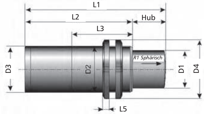
Wellenmutterbefestigung - Fc
