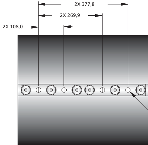
8x Montagebohrungen
