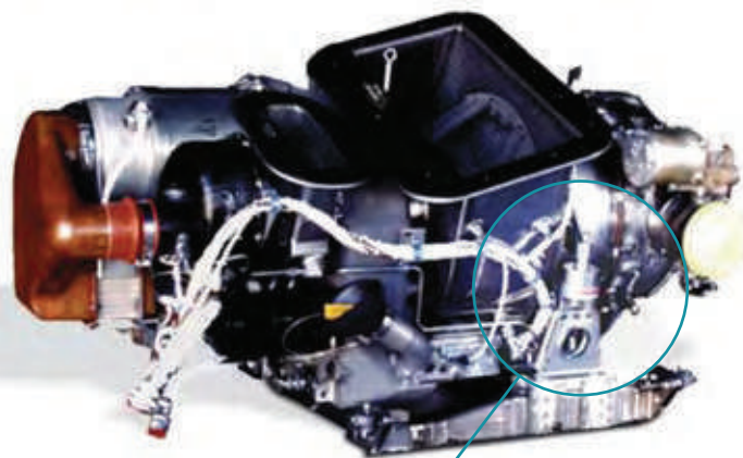
Wire Mesh Isolator (Drahtseildämpfer)
